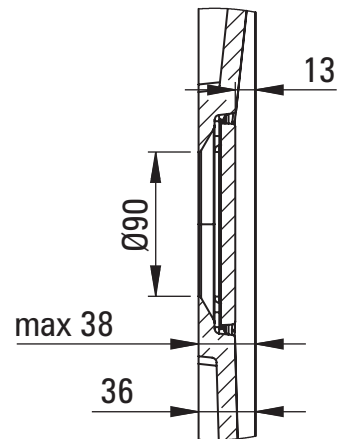
SZCZEGÓŁ B SKALA 1 : 5
