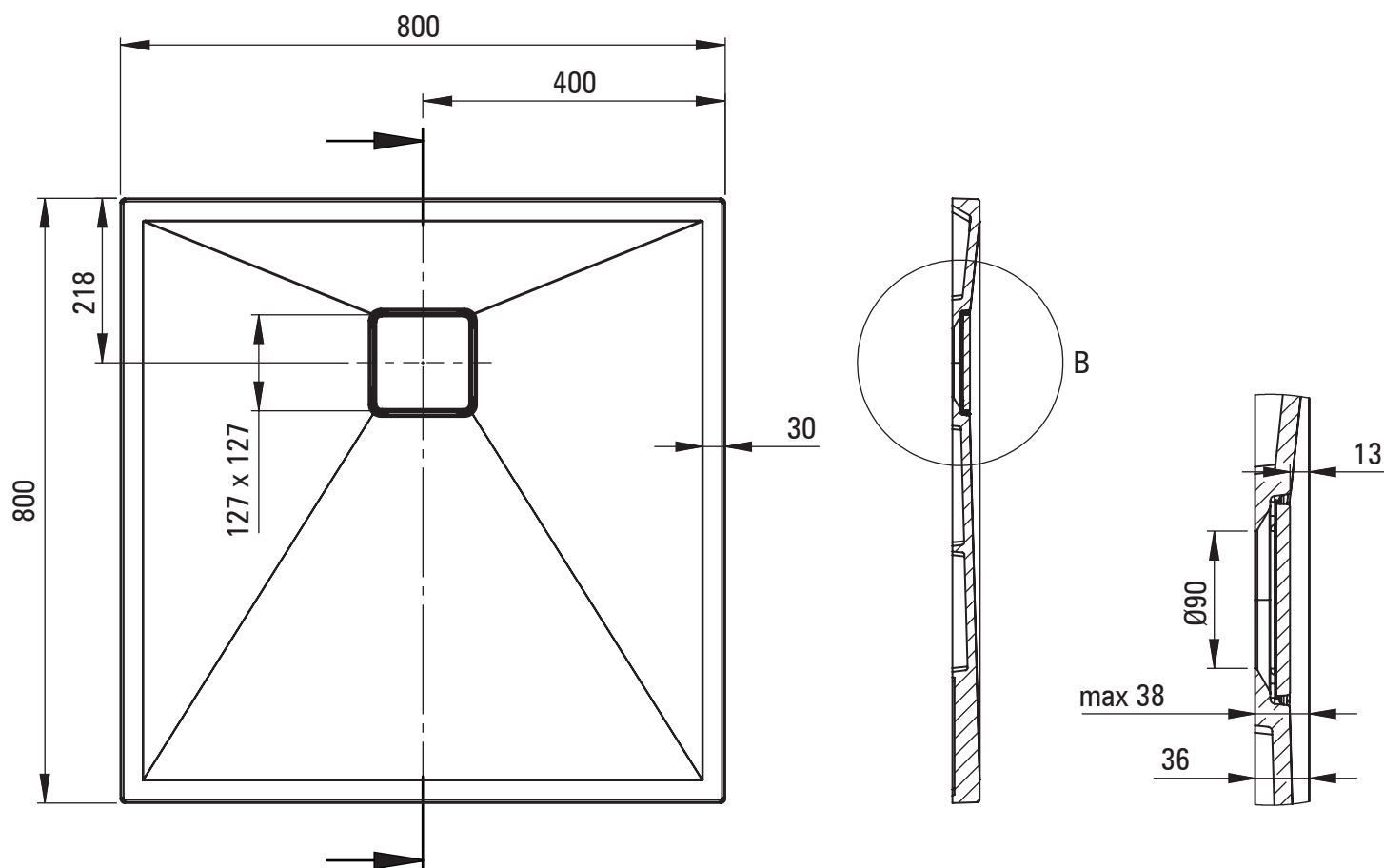
SZCZEGÓŁ B SKALA 1 : 5
